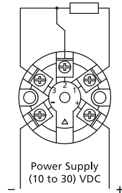
TTR200 Wiring Diagram
